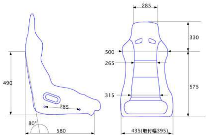
寸法図
